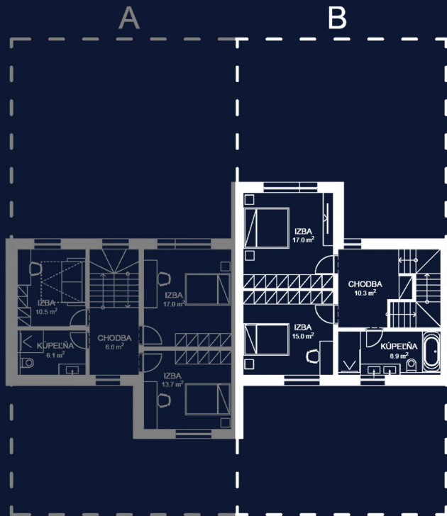
2.NP
