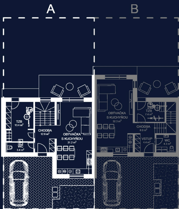
1.NP
